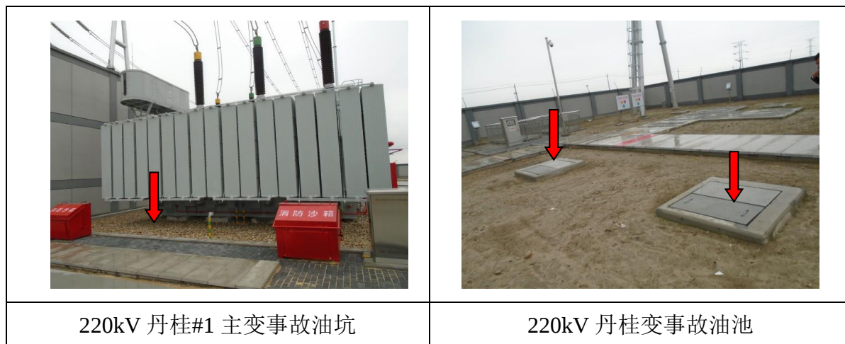
图 6-2 本批验收 220kV 丹桂变电站事故油池照片
