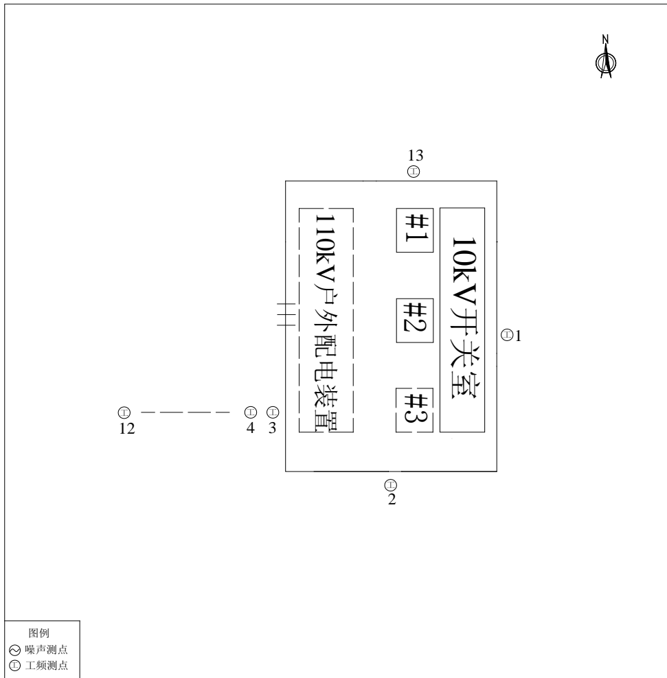
附图 4、110kV 立新变电站（类比站）监测点位示意图
