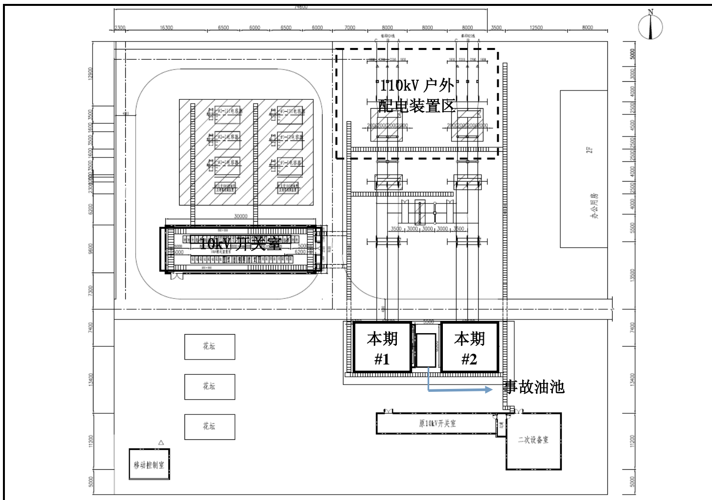
附图 3 110kV 邳州变电站平面布置示意图
