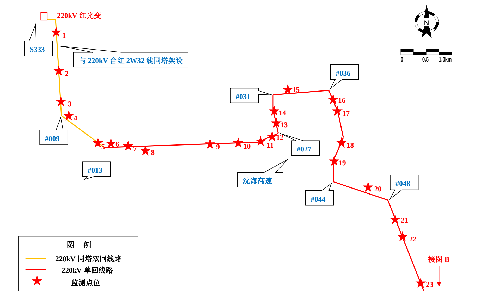
附图 2 东台 220kV 金东变至红光变线路改造工程路径及监测点位示意图 (A)
