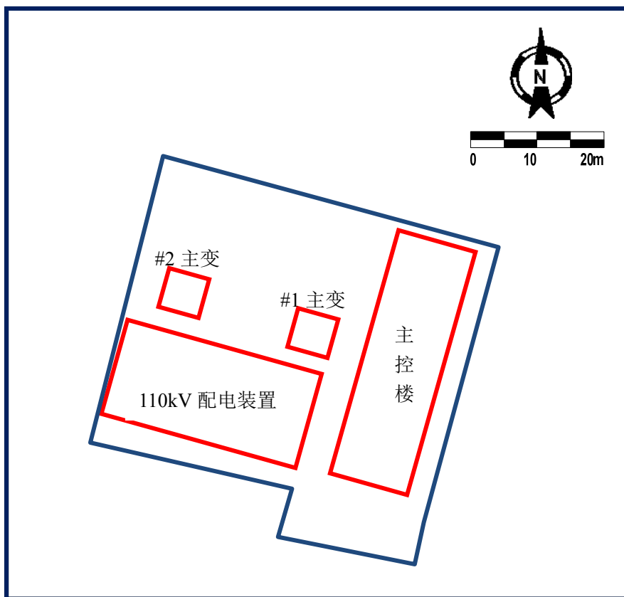
附图 3 田吴 110kV 变电站平面布置图
