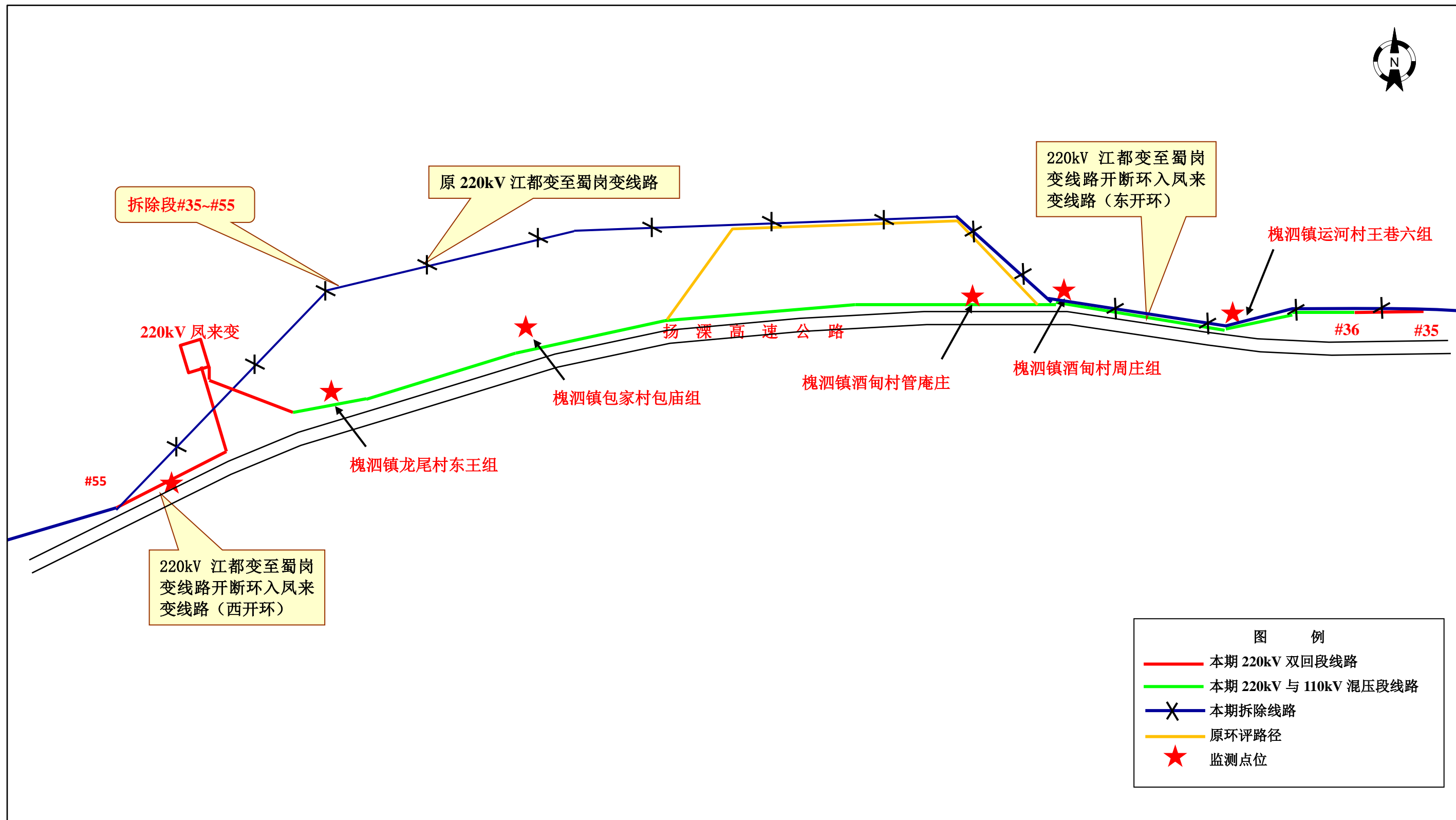
附图 2 220kV 江都变至蜀岗变线路双开断环入凤来变线路工程线路路径示意图
