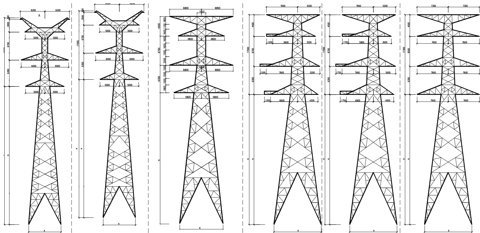
附图3 本工程塔型图
