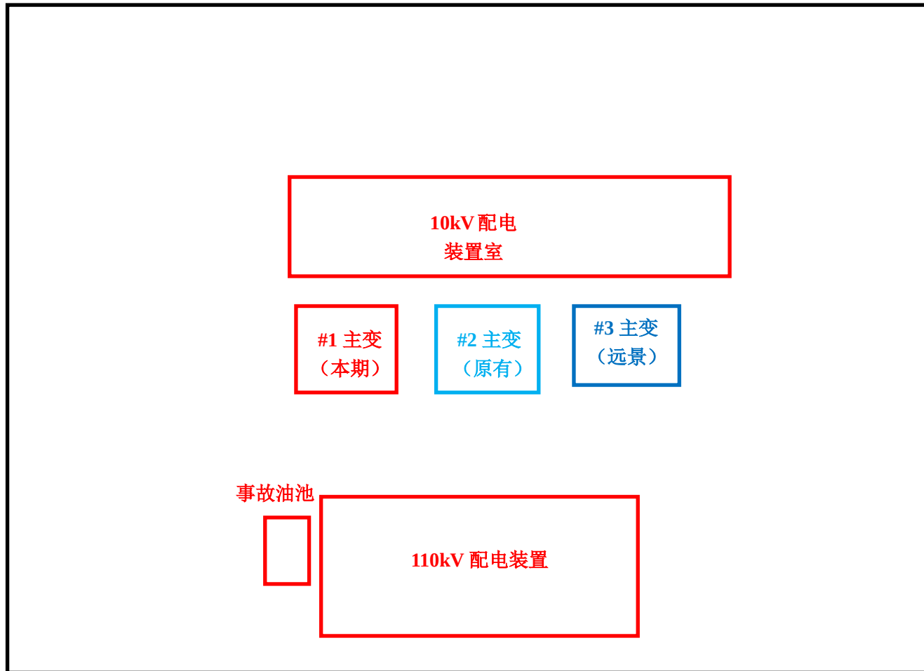
附图 3 110kV 农场变电站总平面布置图
