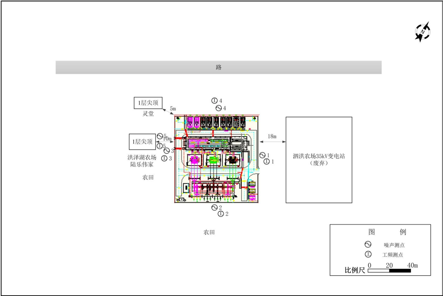
附图 2 110kV 农场变电站监测点位及周围环境示意图
