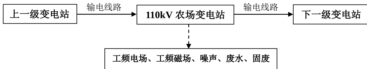
图 1 泗洪 110kV 农场变电站扩建#1 主变工程工艺流程及产污环节示意图
