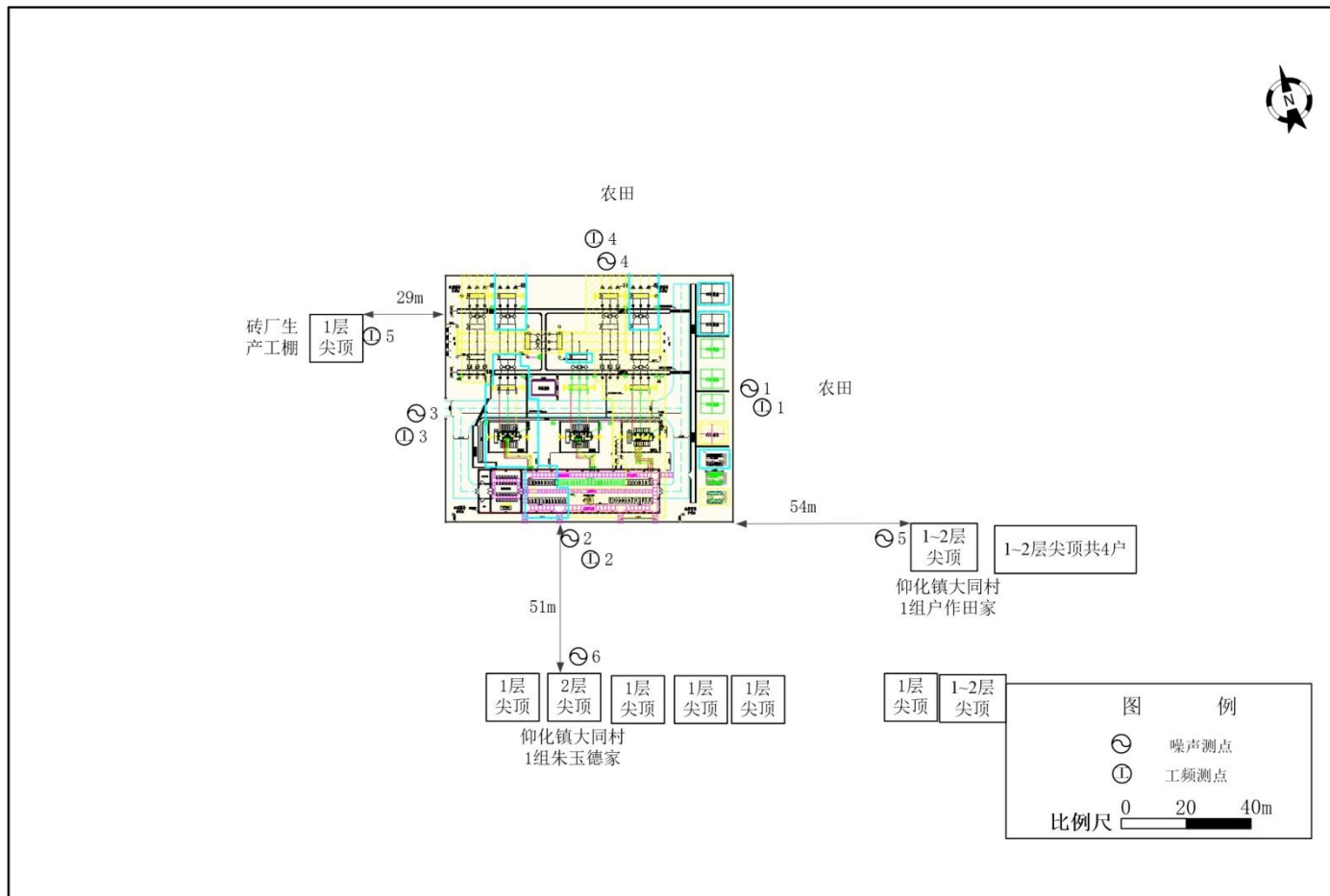
附图 2 110kV 仰化变电站监测点位及周围环境示意图
