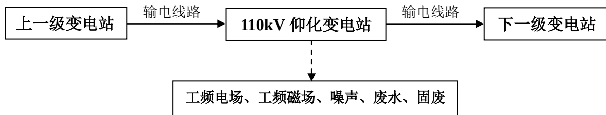
图 1 宿迁 110kV 仰化变电站扩建#3 主变工程工艺流程及产污环节示意图
