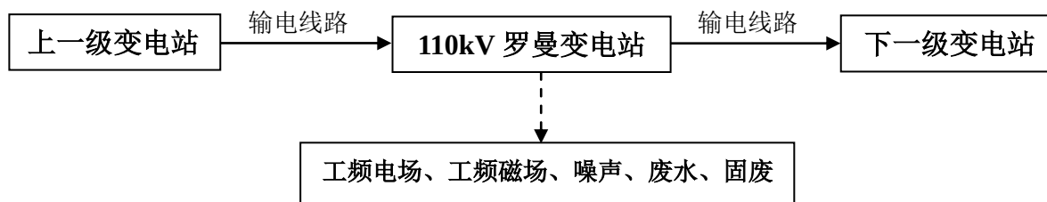
图 1 宿迁 110kV 罗曼变电站扩建#2 主变工程工艺流程及产污环节示意图
