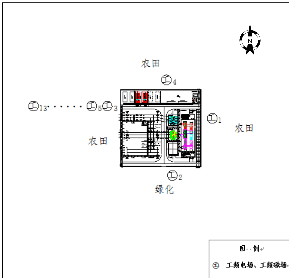
附图 4 110kV 练湖变电站（类比站）监测点位示意
