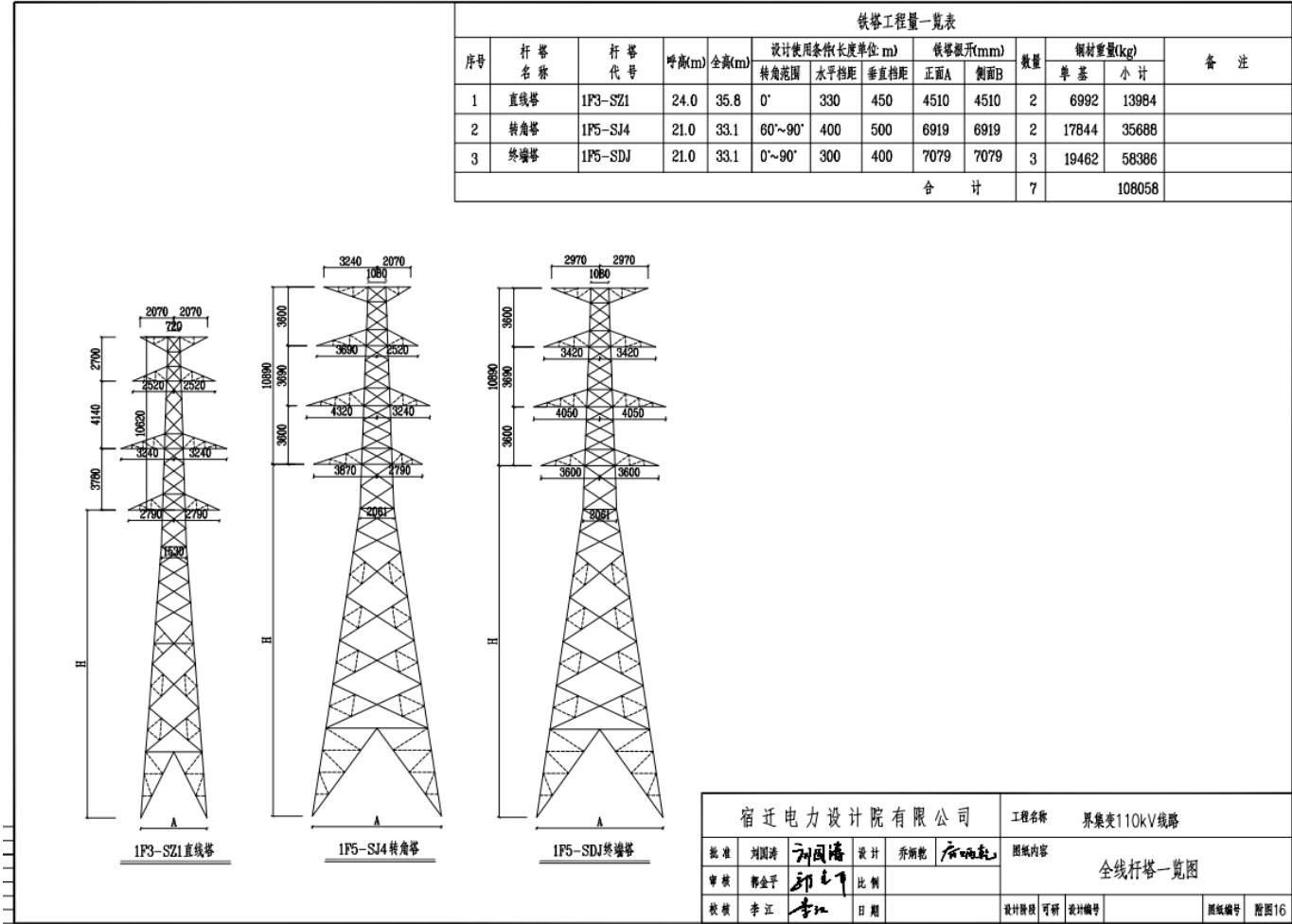
附图 6 本工程塔型图
