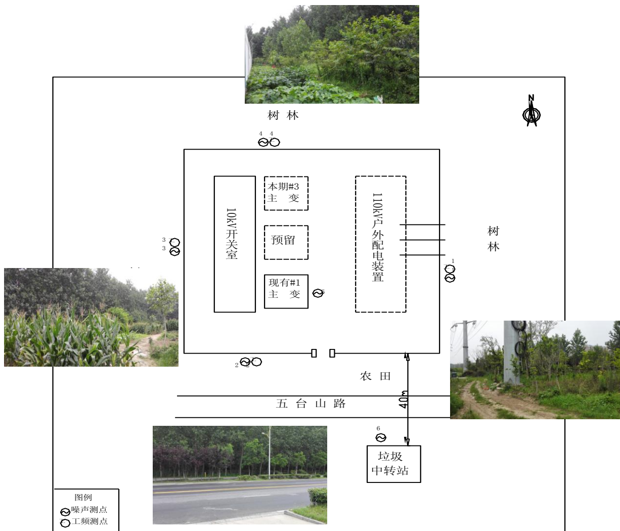
附图 2 110kV 豫东变电站监测点位及周围环境示意图
