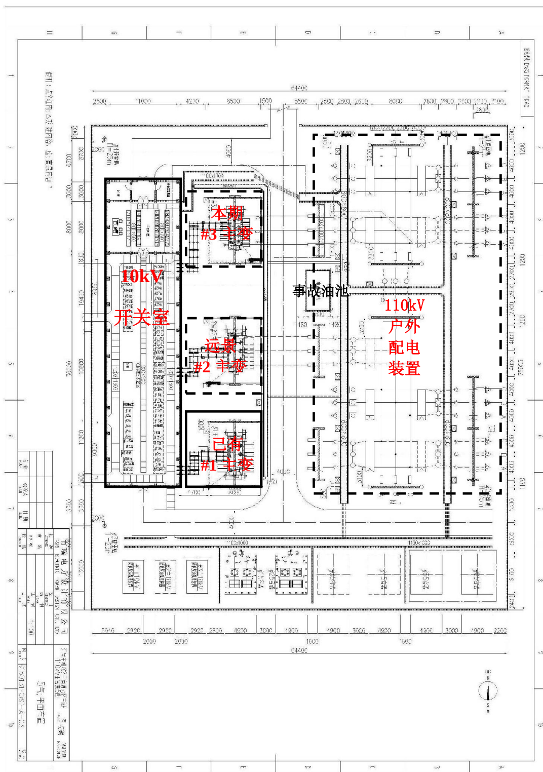
附图 3 110kV 王官集变电站平面布置示意图
