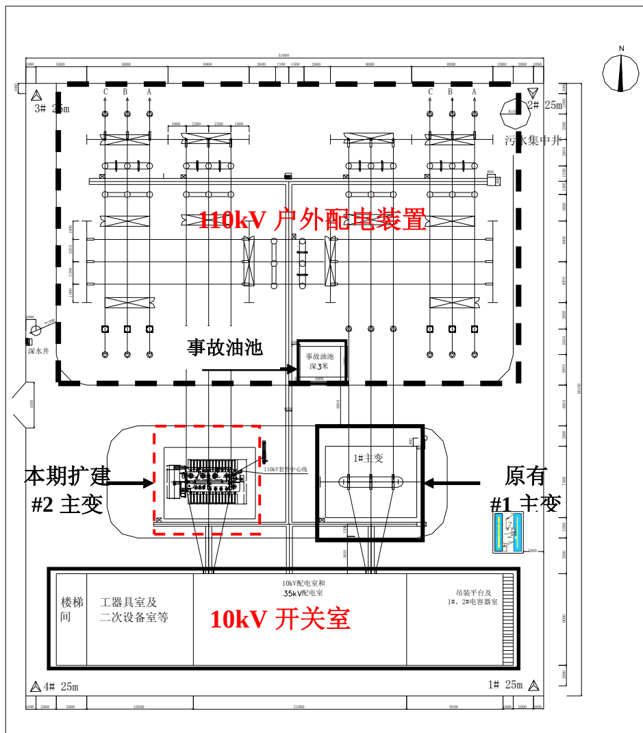
附图3 110kV 埤子变电站平面布置示意图
