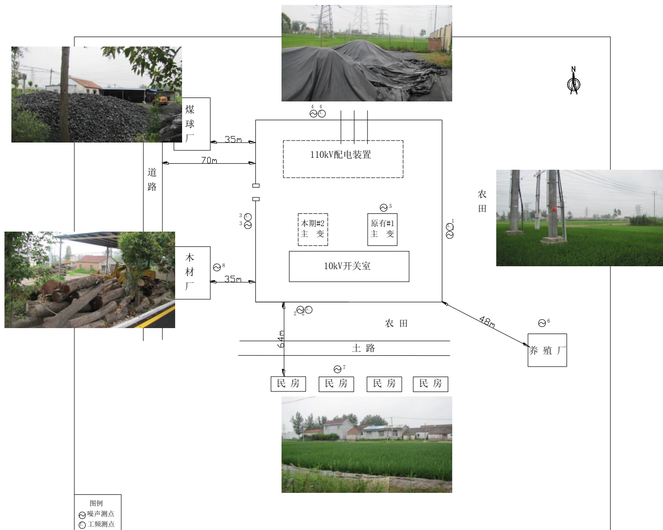
附图 2 110kV 埤子变电站监测点位及周围环境示意图
