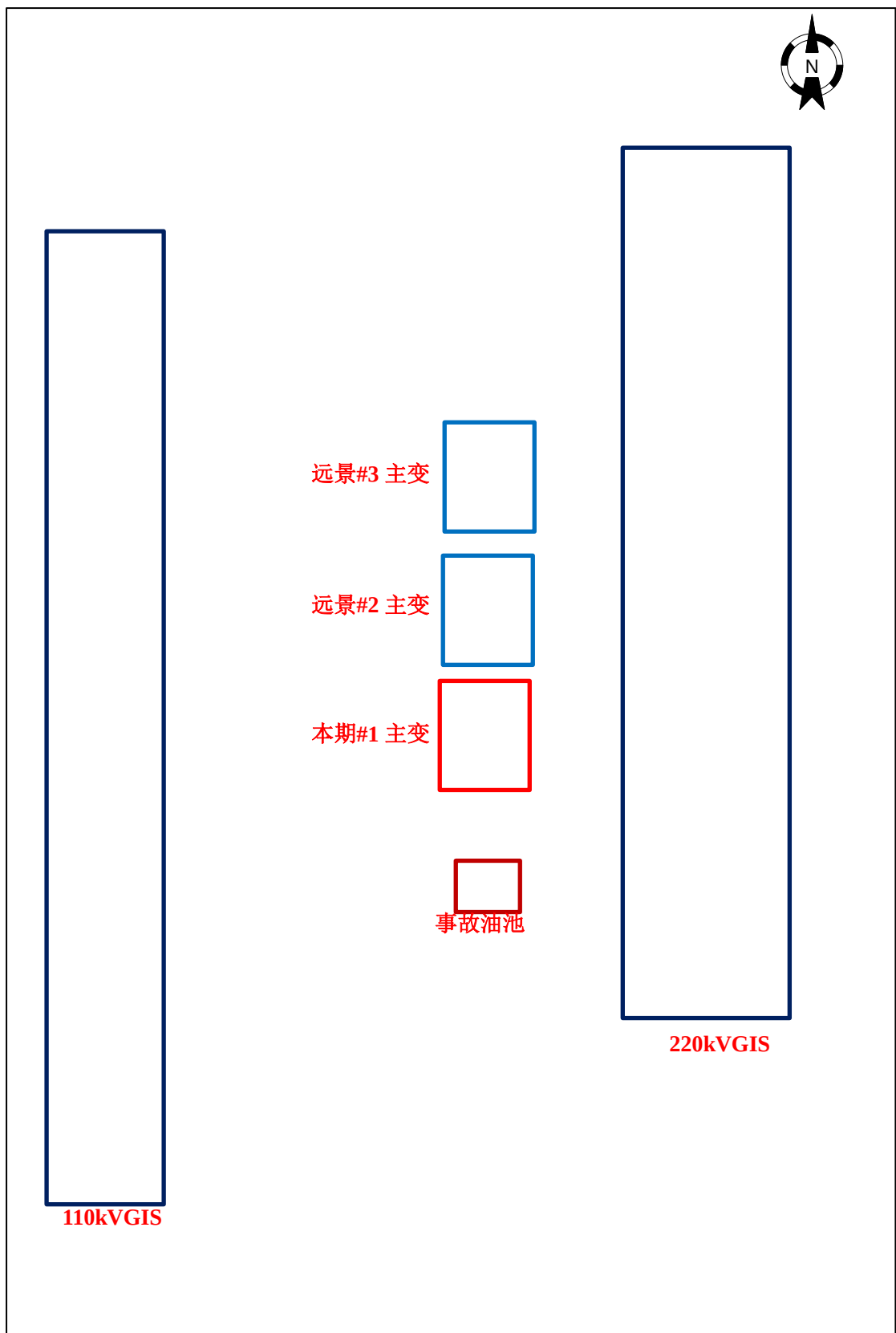
附图 3 童画 220kV 变电站平面布置图
