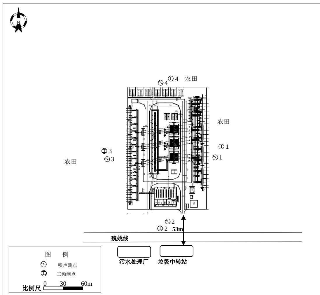
附图 2 童画 220kV 变电站拟建址周围监测点位及环境示意图
