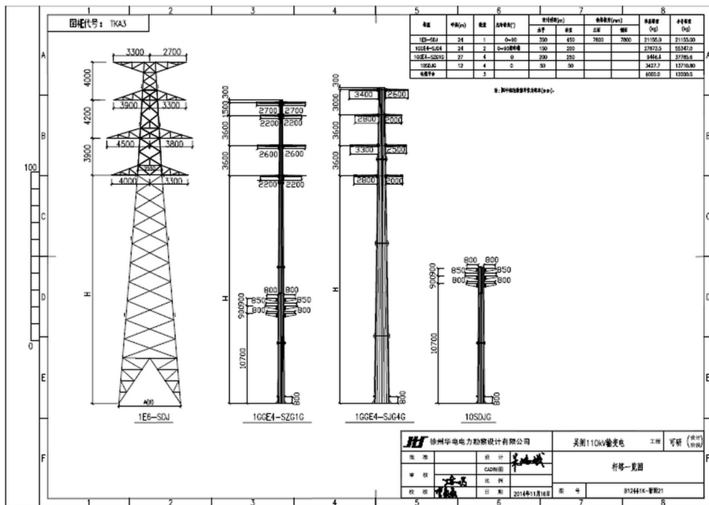
附图 5、110kV 吴闸变配套 110kV 线路杆塔图
