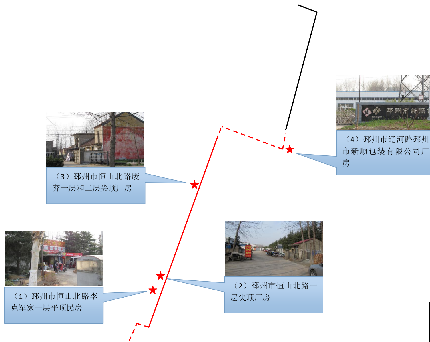
附图 4、110kV 吴闸变配套 110kV 线路路径及监测点位示意图
