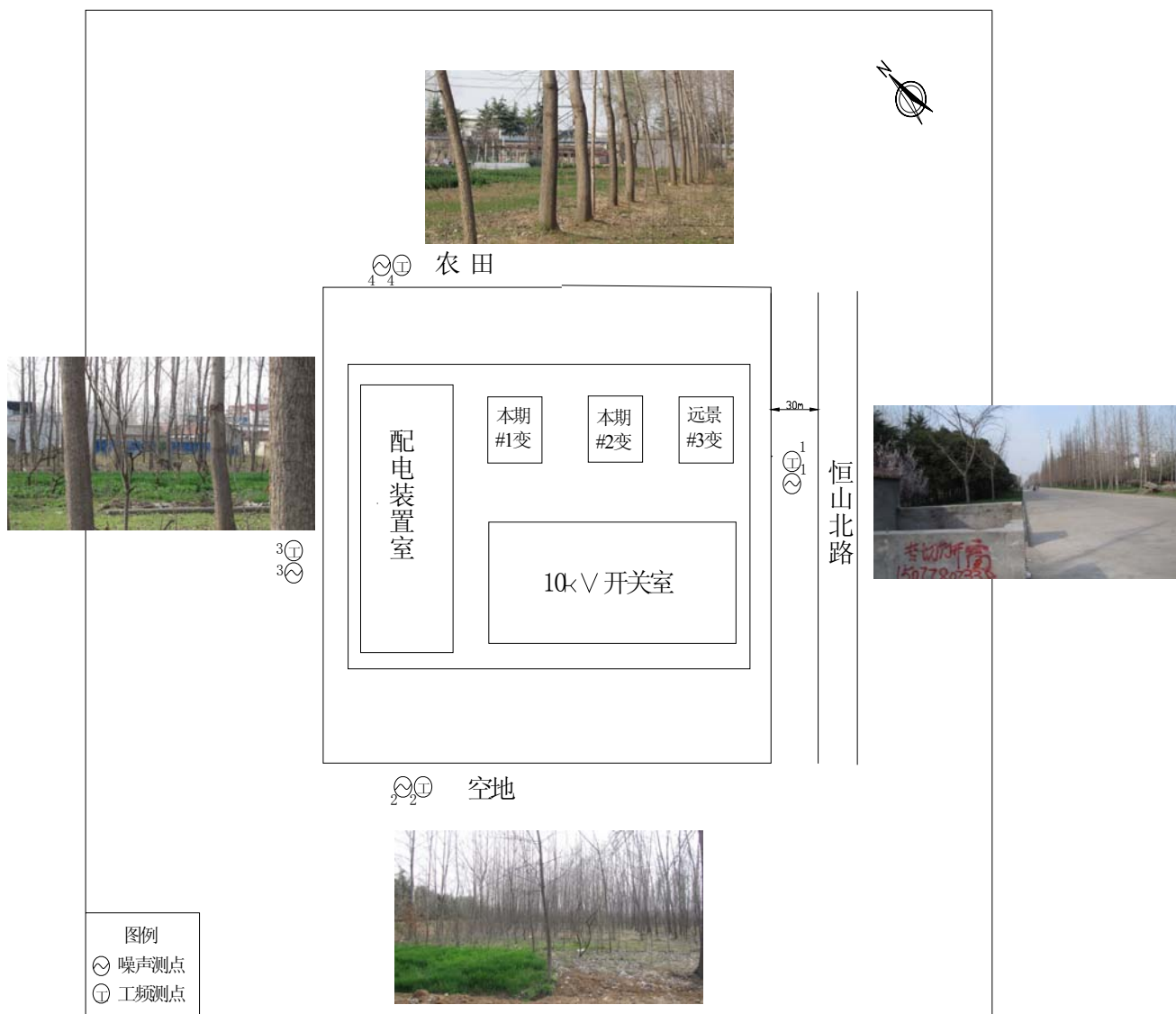
附图 2、邳州 110kV 吴闸变监测点位布置示意图
