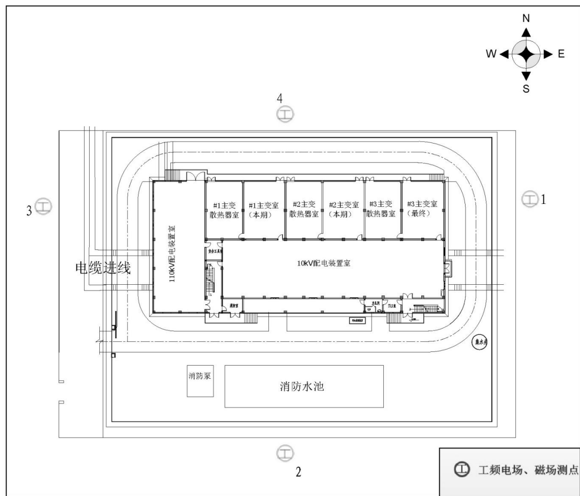
附图 6、110kV 句北变电站（类比站）监测点位示意图
