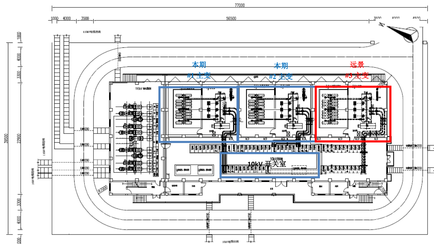
附图 3、110kV 吴闸变平面布置示意图
