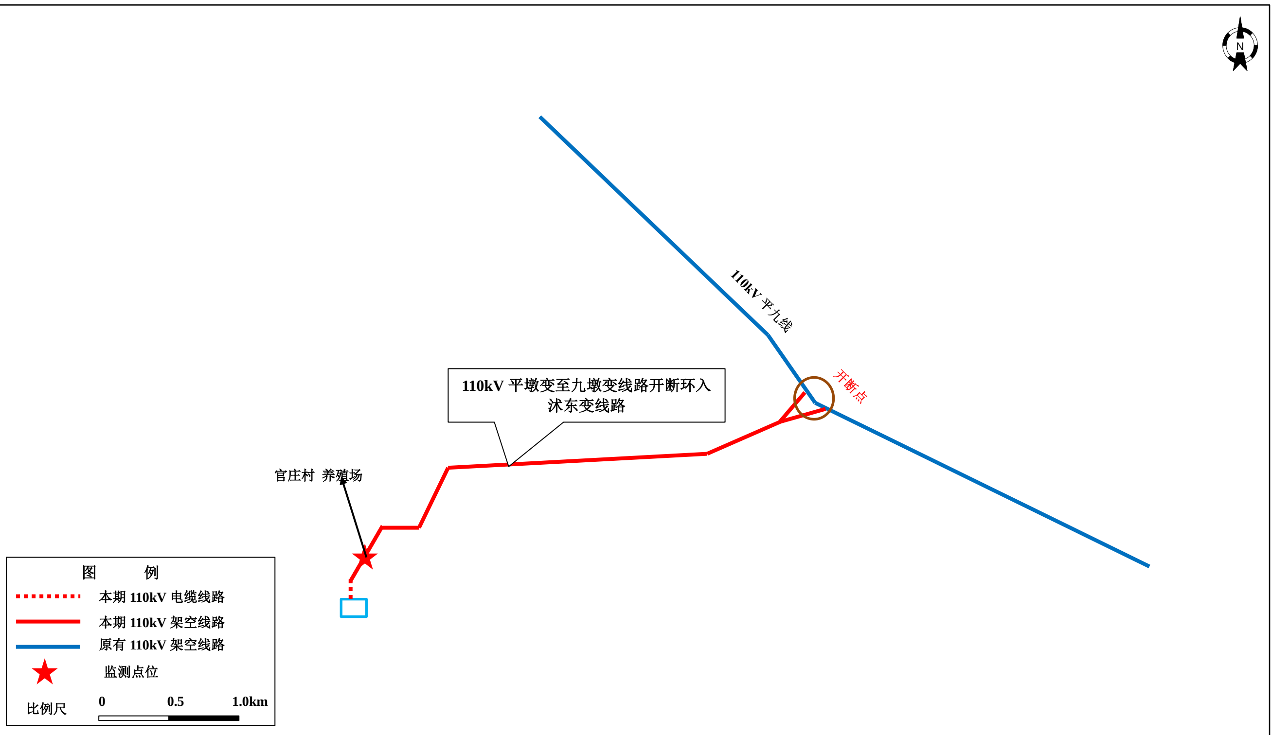
附图 4 110kV 线路路径及监测点位示意图 (a)
