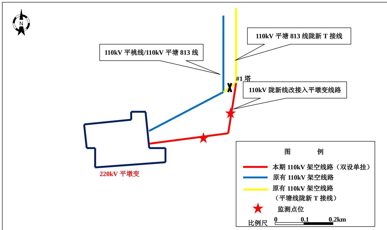
附图 4 110kV 线路路径及监测点位示意图 (b)
