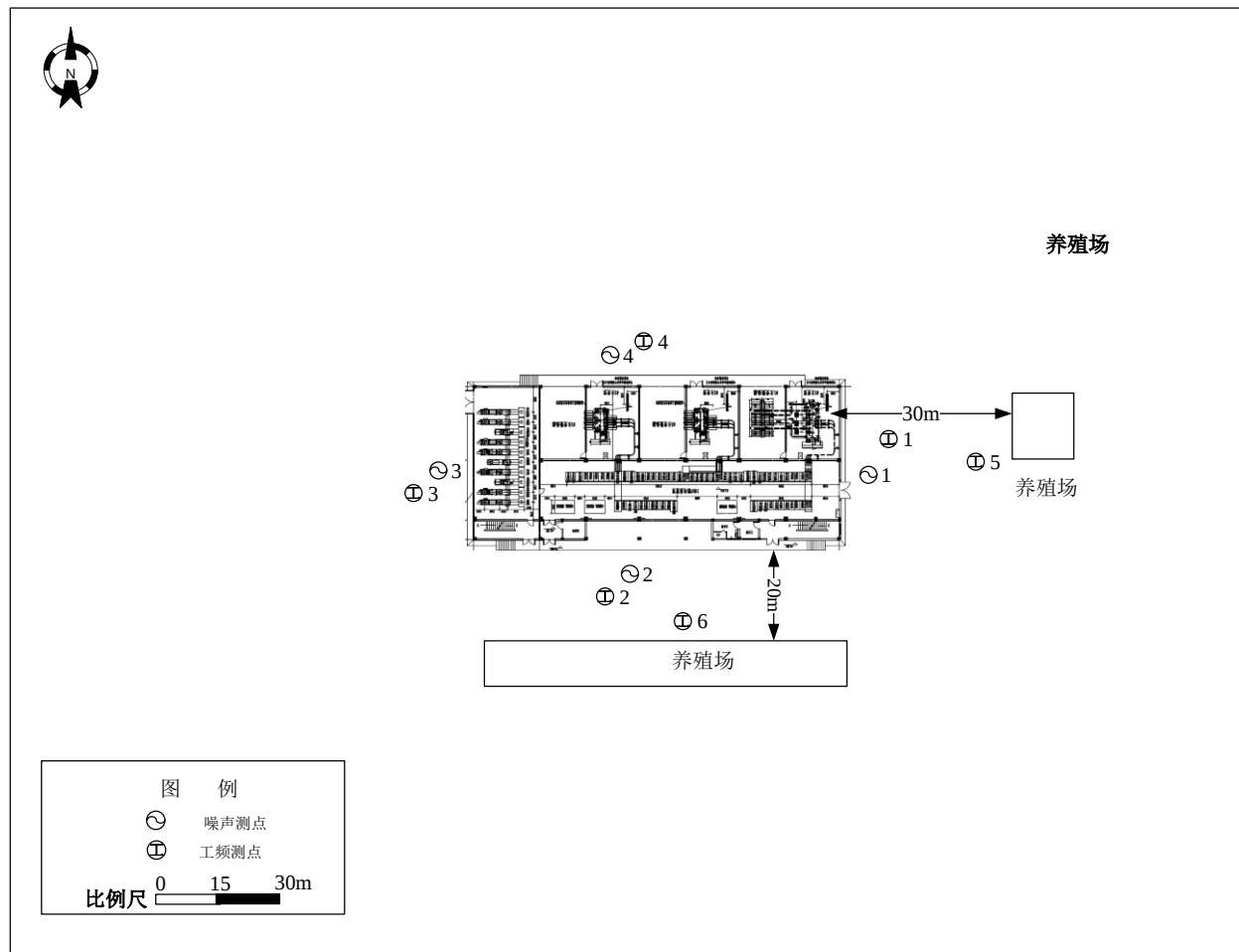
附图 2 110kV 沐东变电站拟建址周围监测点位及环境示意图
