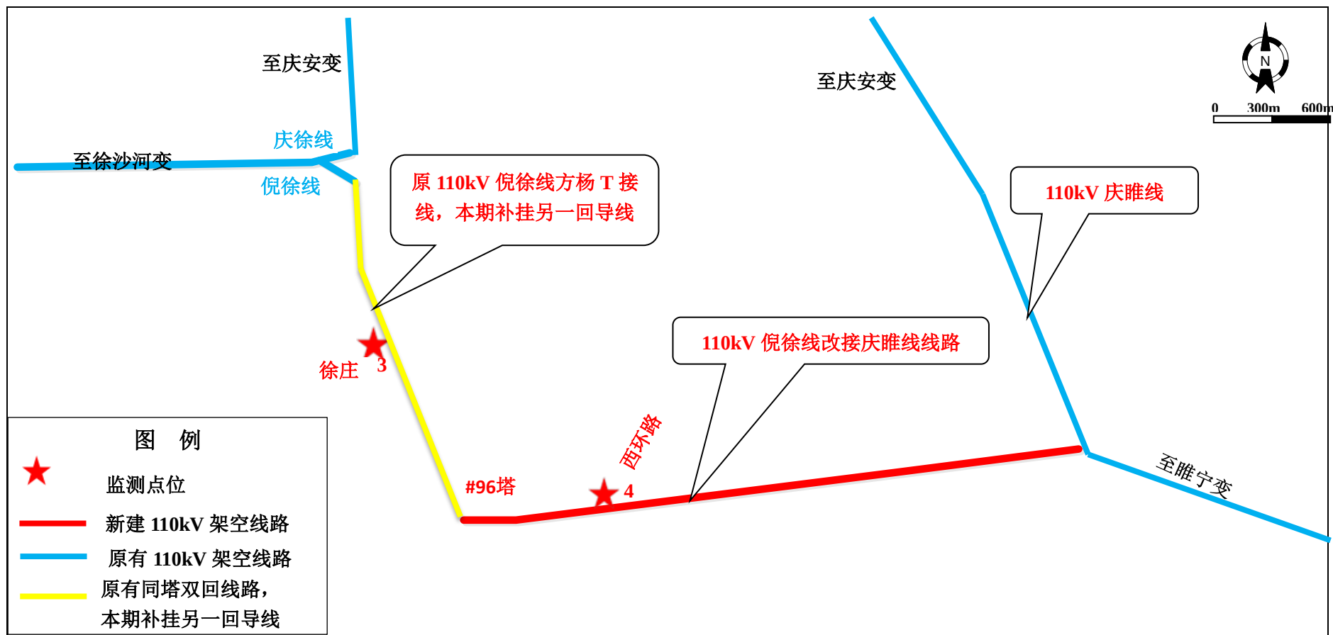
附图 2 睢宁 220kV 子仙变 110kV 配套线路工程线路路径及监测点位示意图 (c)
