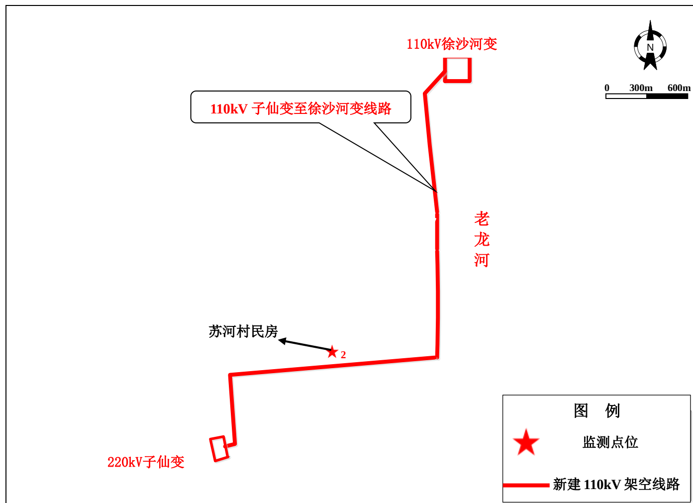
附图 2 睢宁 220kV 子仙变 110kV 配套线路工程线路路径监测点位示意图 (b)
