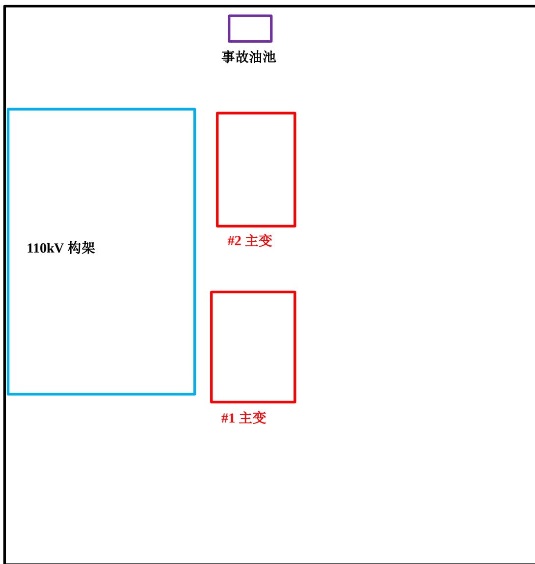
附图 3 110kV 统一变电站平面布置图
