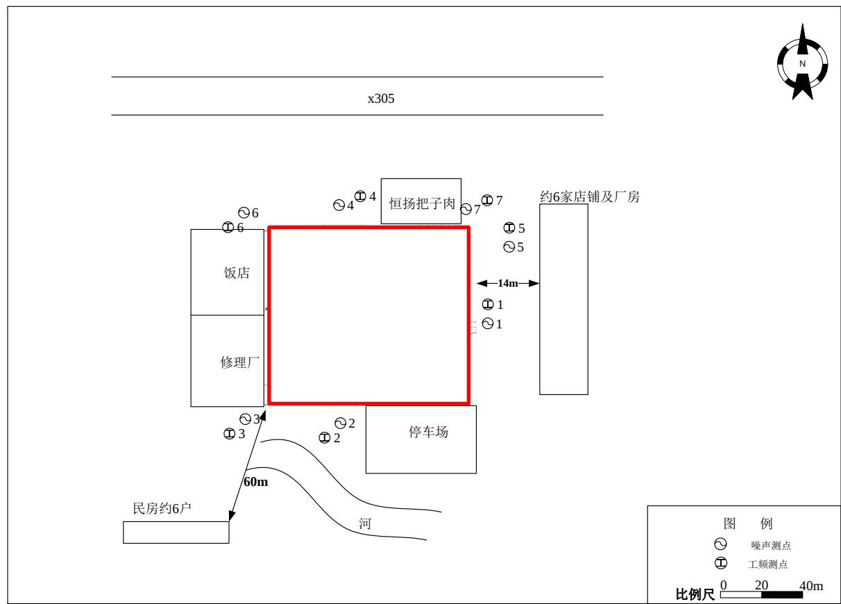
附图 2 110kV 孙庄变电站检测点位及周围环境示意图
