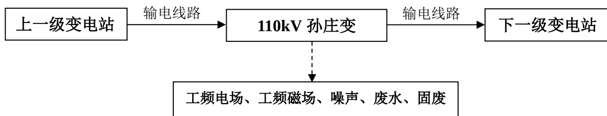
图 1 110kV 孙庄变#2 主变增容工程工艺流程及产污环节示意图
