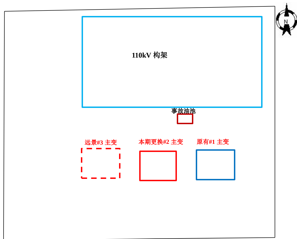
附图 3 110kV 孙庄变电站总平面布置图
