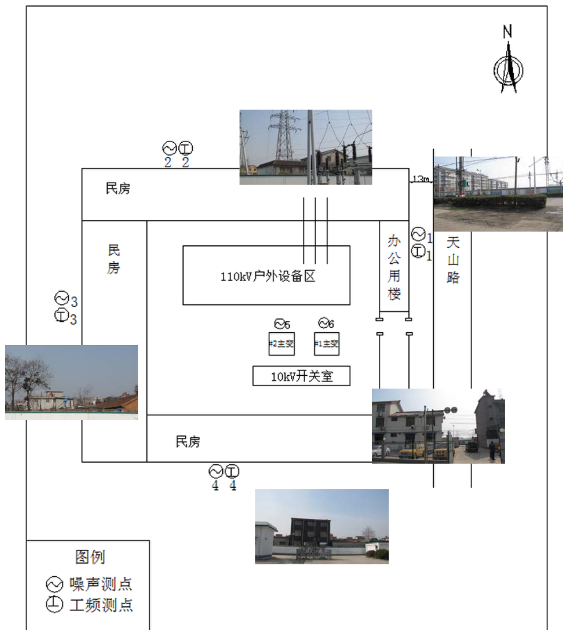
附图 2 110kV 邳州变电站监测点位及周围环境示意图
