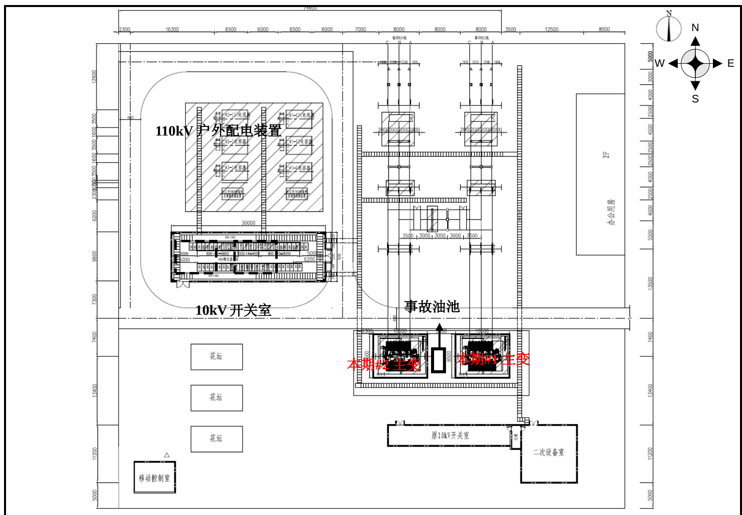
附图 3 110kV 邳州变平面布置示意图
