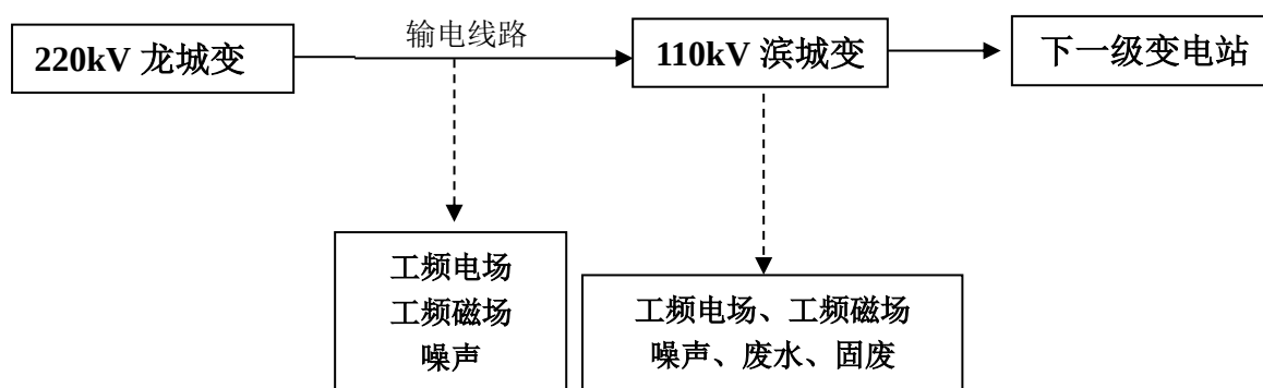
图 1 110kV 输变电工程工艺流程及产污环节示意图
