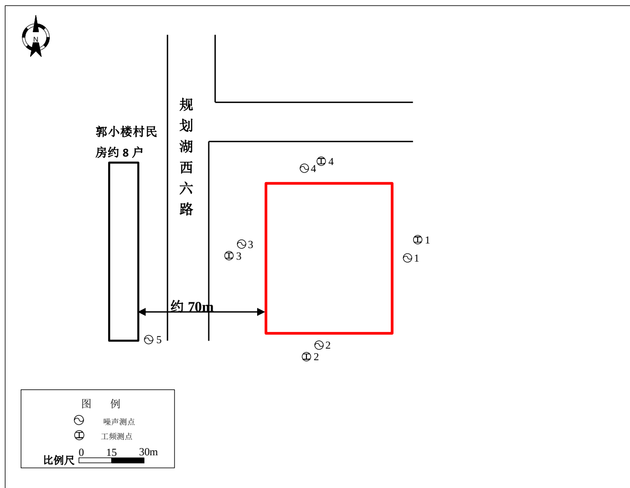
附图2 110kV 滨城（东关）变电站拟建址周围监测点位及环境示意图
