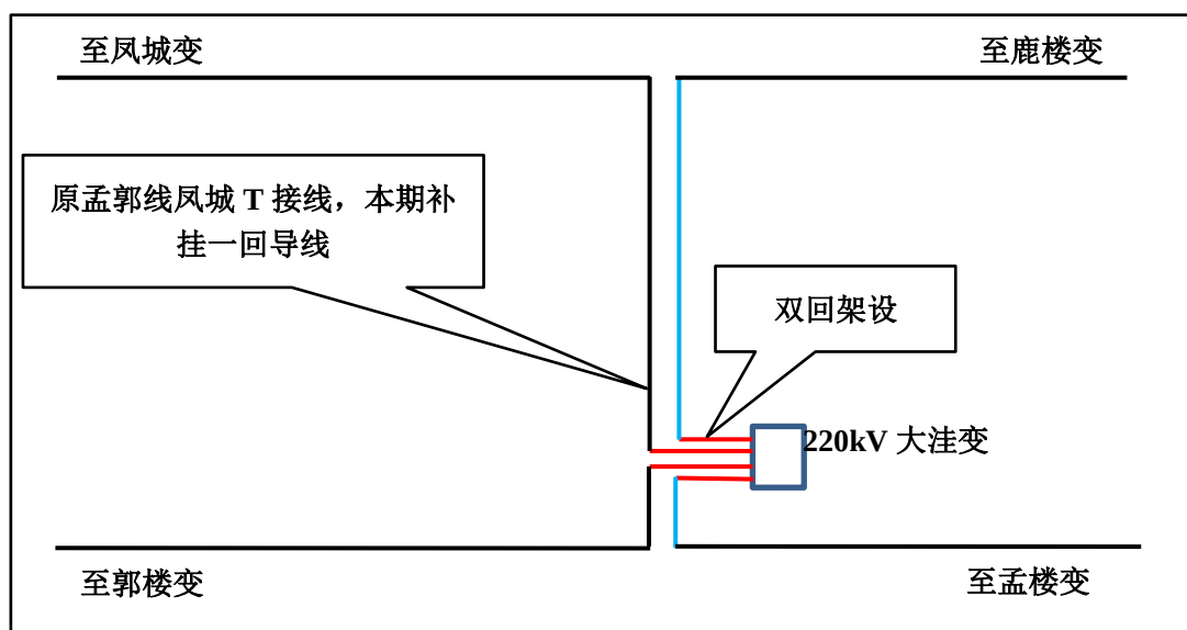
本工程接线示意图
