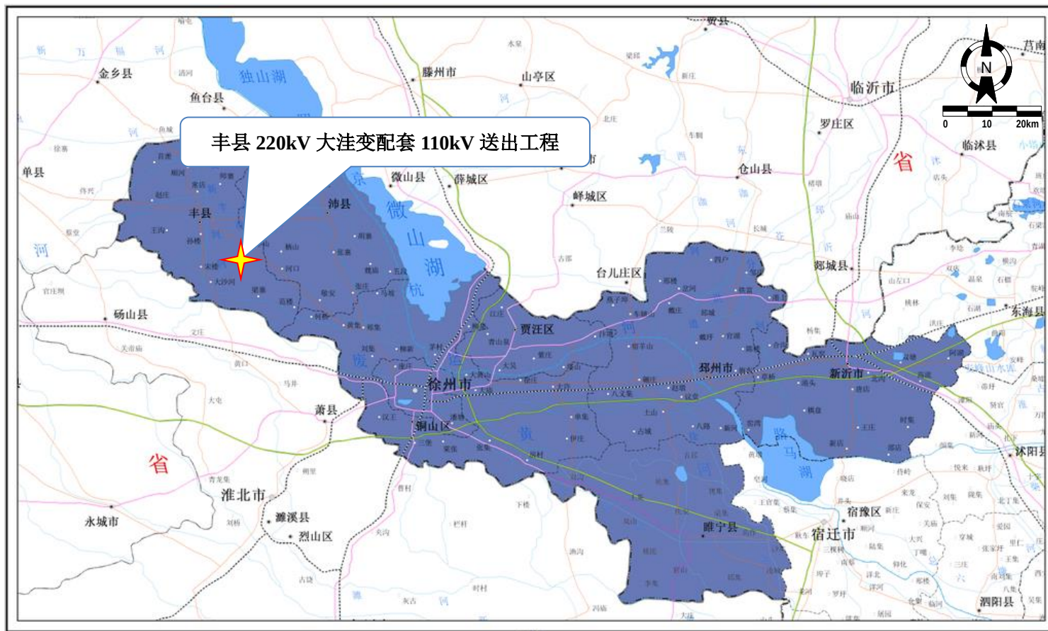
附图 1 丰县 220kV 大洼变配套 110kV 送出工程地理位置示意图
