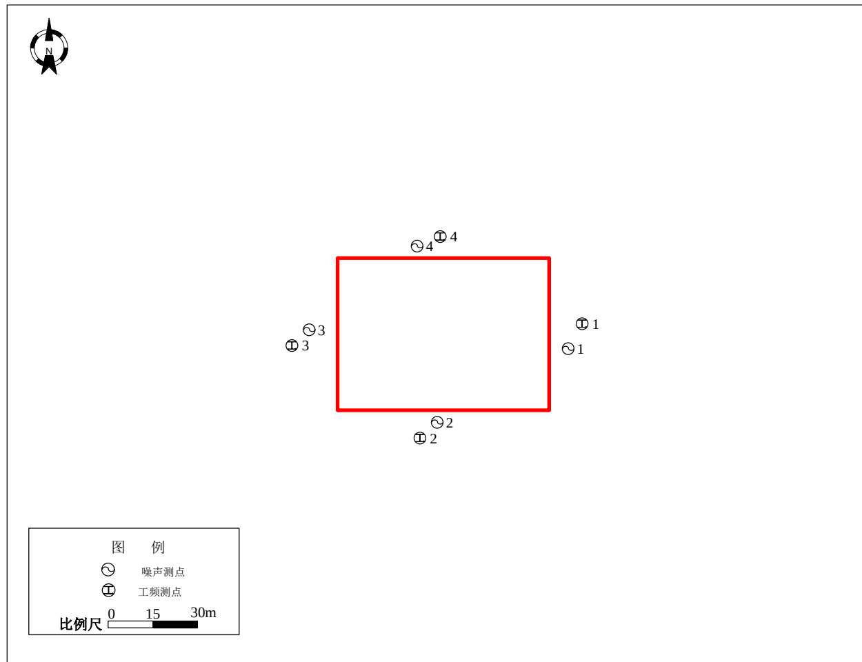
附图 2 110kV 大沙河（李寨）变电站拟建址周围监测点位及环境示意图
