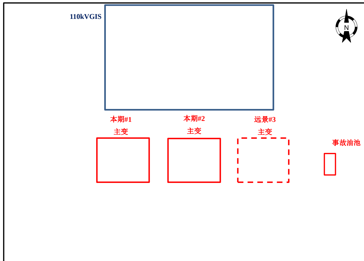
附图3 110kV 大沙河（李寨）变平面布置示意图
