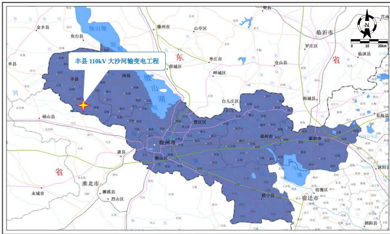
附图 1 丰县 110kV 大沙河（李寨）输变电工程地理位置示意图
