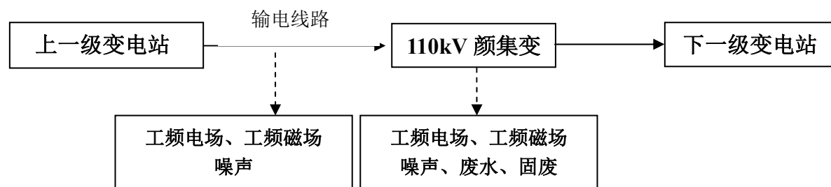
图 2 110kV 输变电工程工艺流程及产污环节示意图
