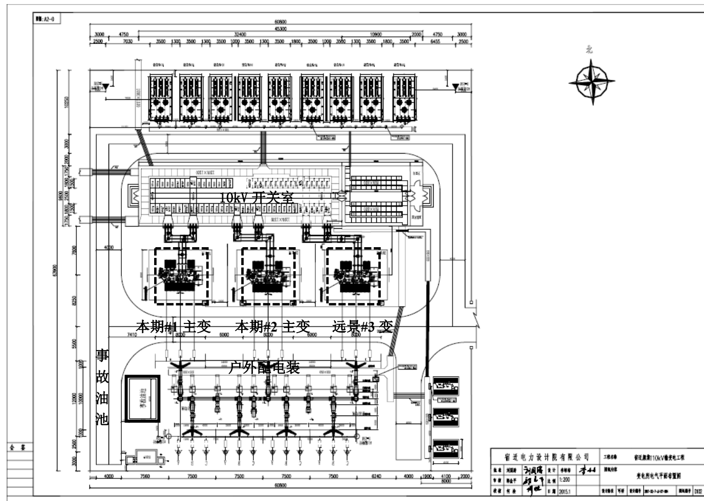
附图 3、110kV 颜集变平面布置示意图
