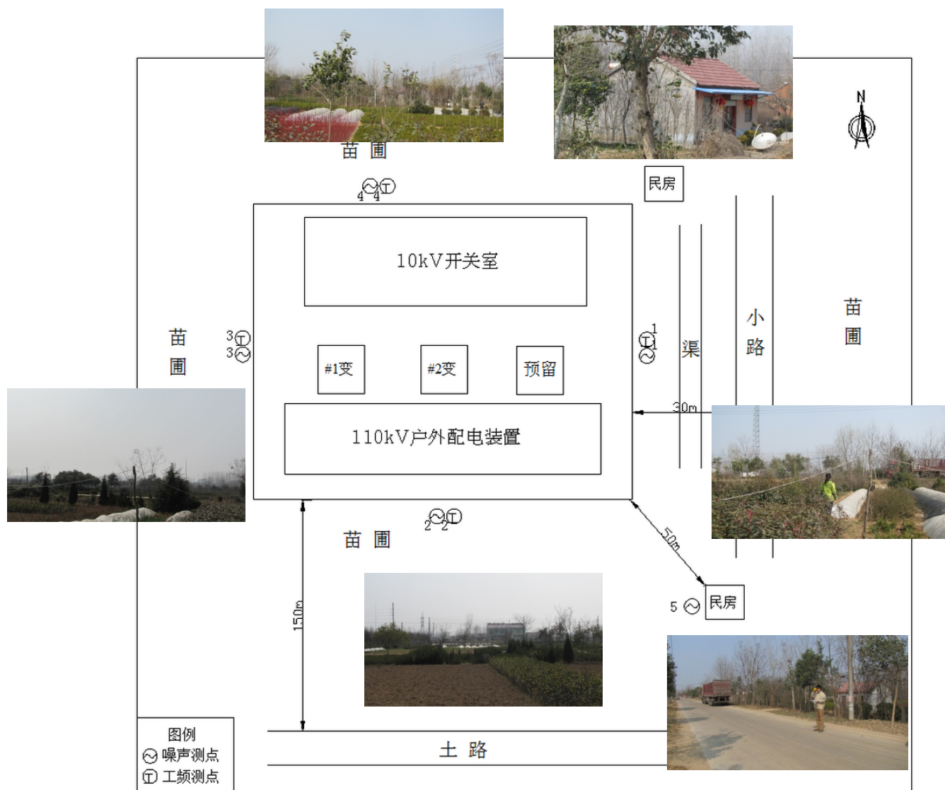
附图 2、110kV 颜集变监测点位及周围环境示意图
