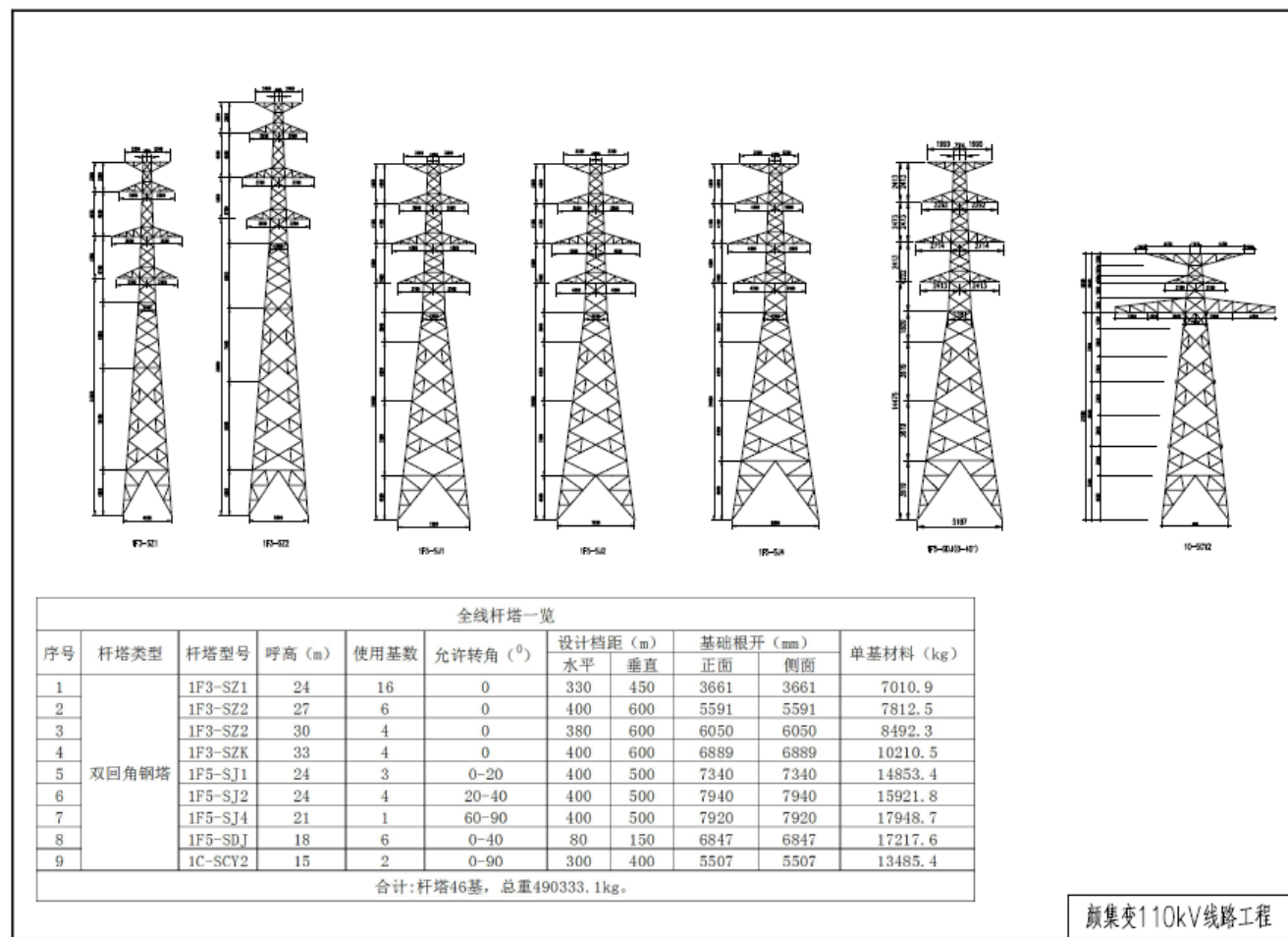
附图 5、110kV 颜集变配套 110kV 线路杆塔图
