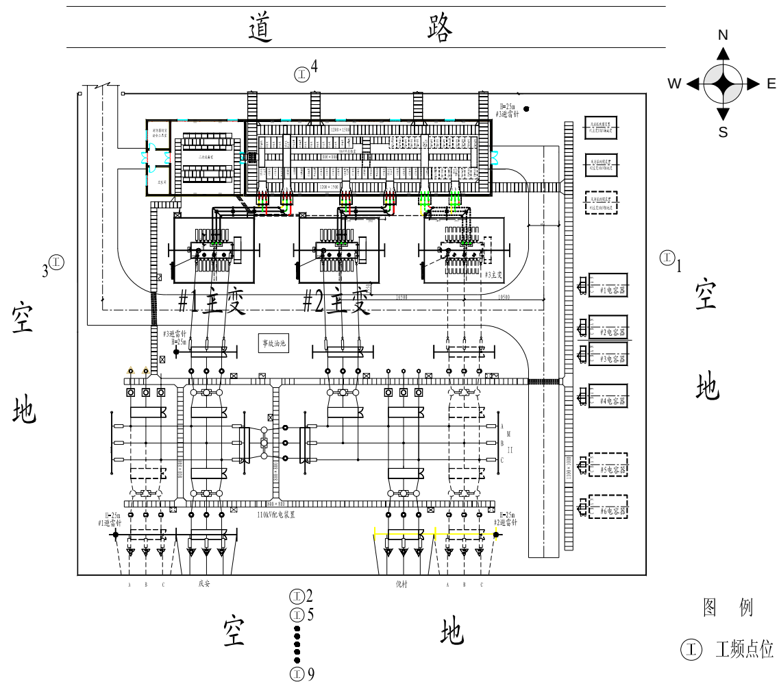
附图 8、110kV 联群变电站（类比站）监测点位示意图
