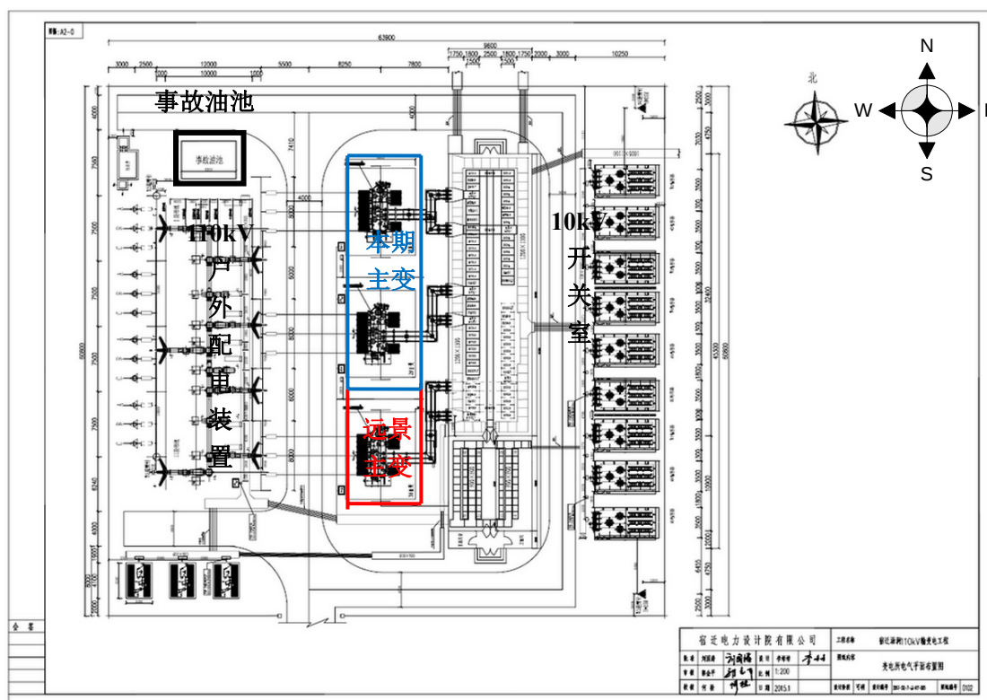
附图 3、110kV 汤润变平面布置示意图
