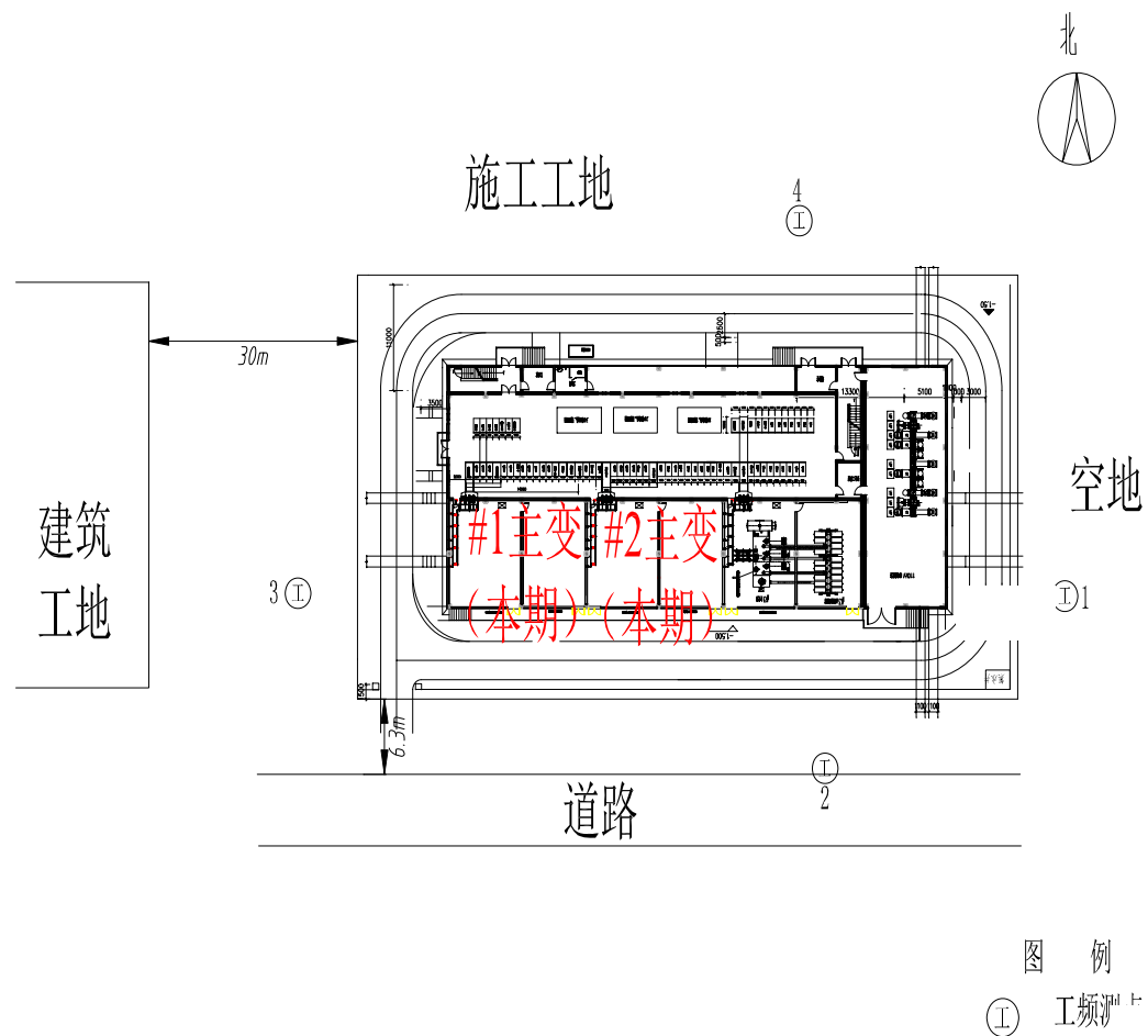
附图 4 110kV 禹山变电站（类比站）监测点位示意图
