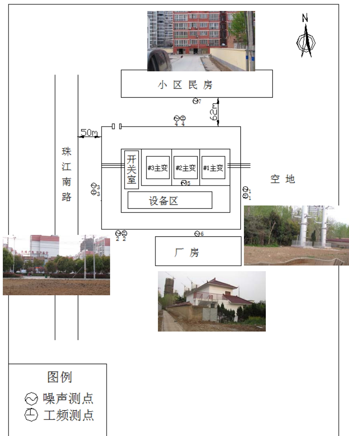
附图2 110kV 花乡变电站监测点位及周围环境示意图
