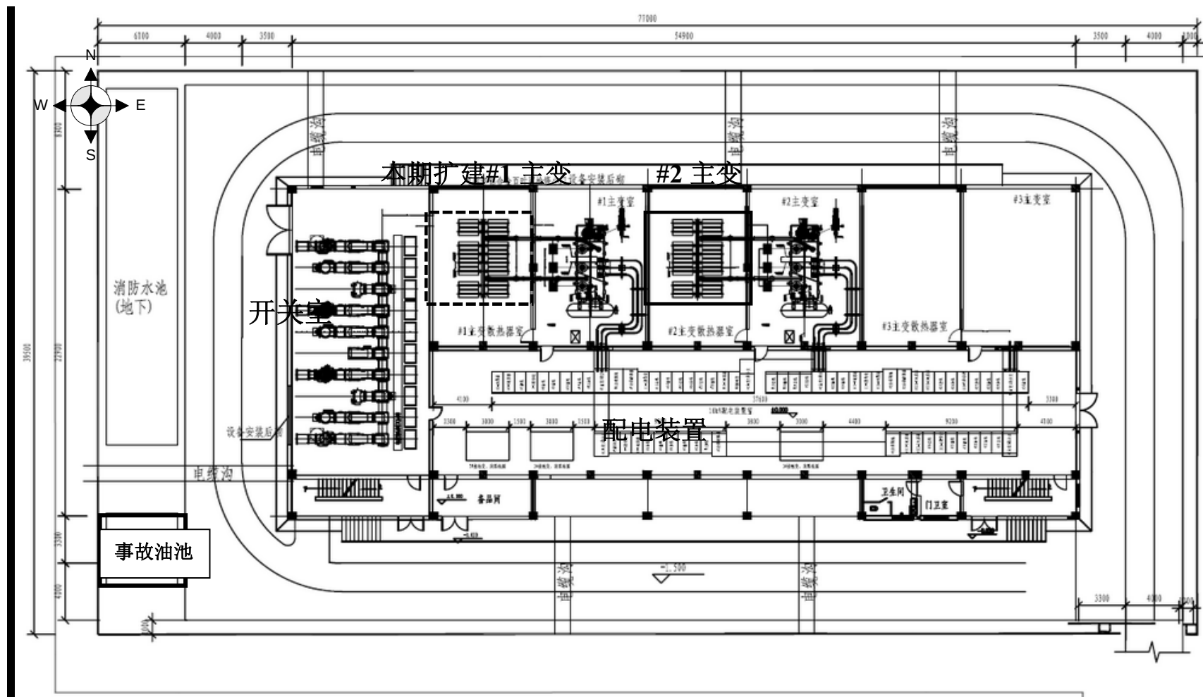
附图 3 110kV 花乡变平面布置示意图
