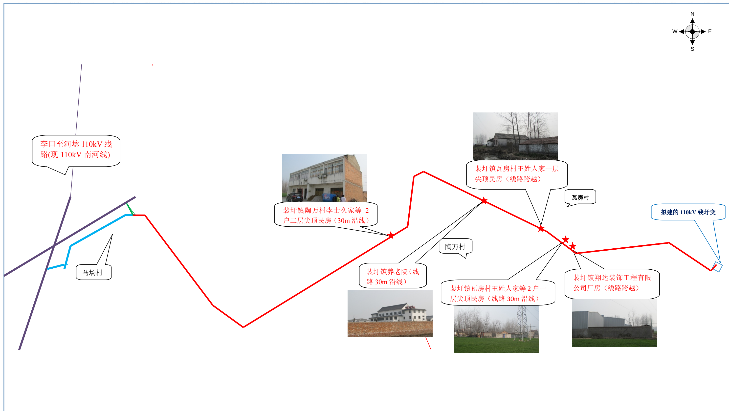
附图 5、110kV 裴圩变配套 110kV 线路路径及监测点位示意图
