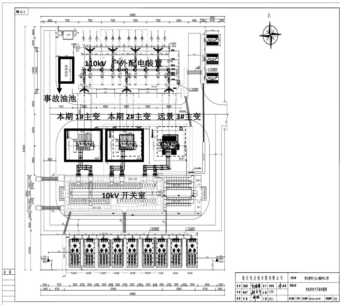
附图 3、110kV 裴圩变平面布置示意图
