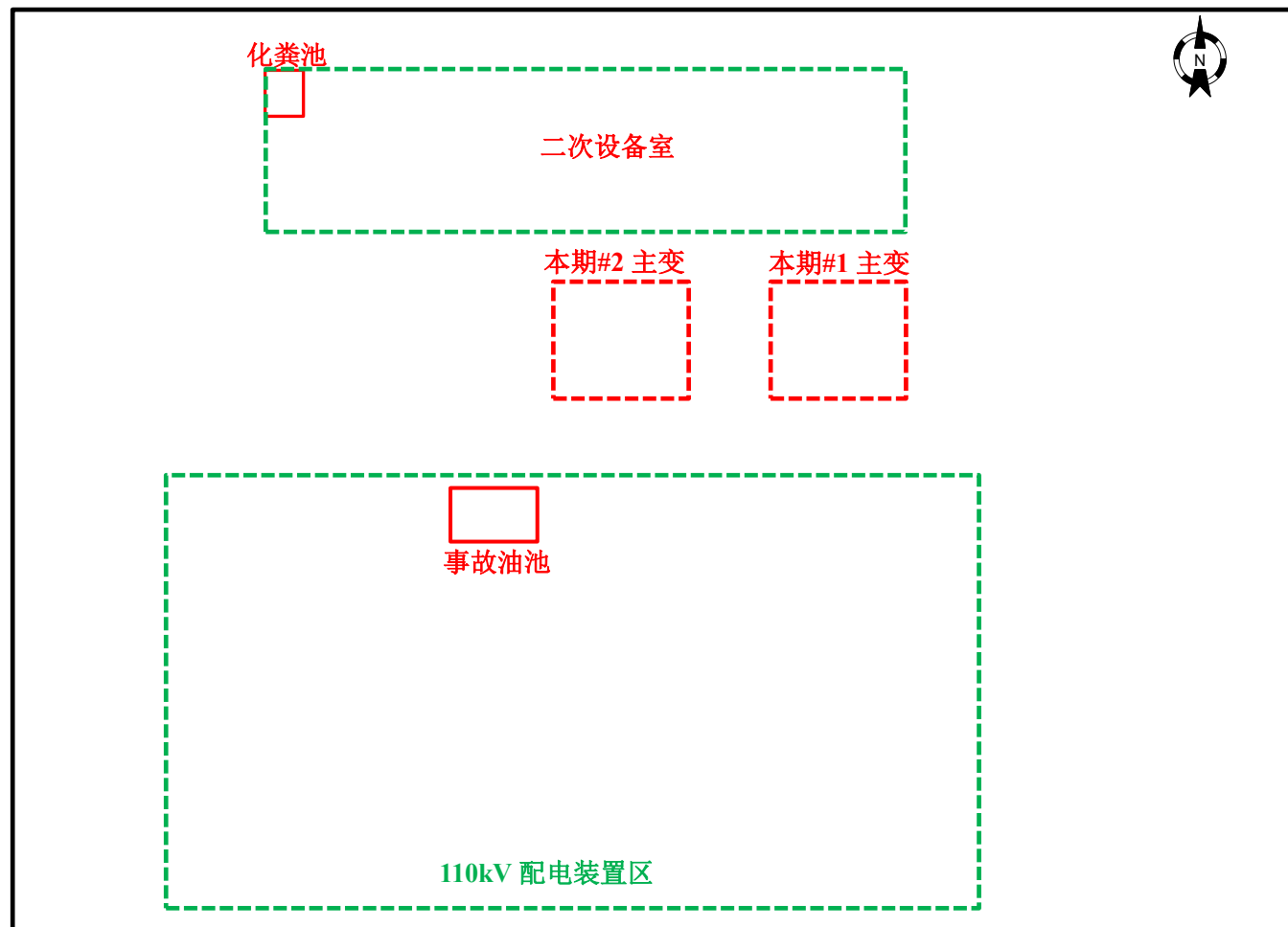
附图 3 110kV 龙河变电站平面布置示意图
